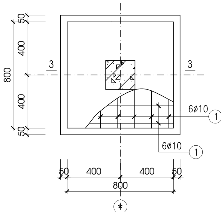
MÓNG M1 (SL: 02)
