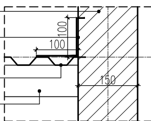
Chi tiết liên kết mái tôn và tường
